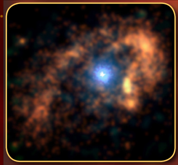
Eta Carinae
