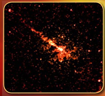
Centaurus A
